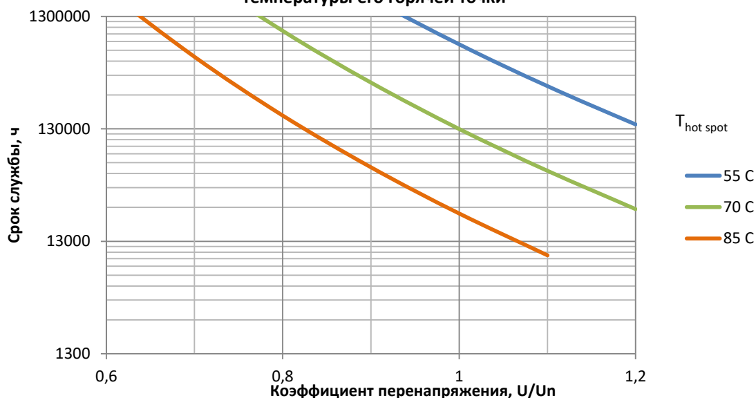
Зависимость ожидаемого срока службы конденсатора от напряжения и температуры его горячей точки
